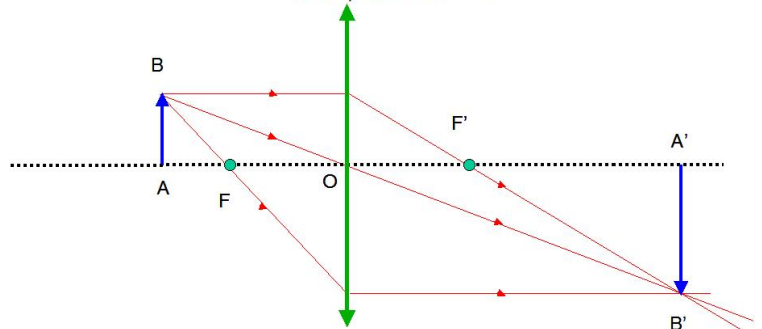
Objet situé à une distance d de la lentille telle que OF < d < 2 OF
