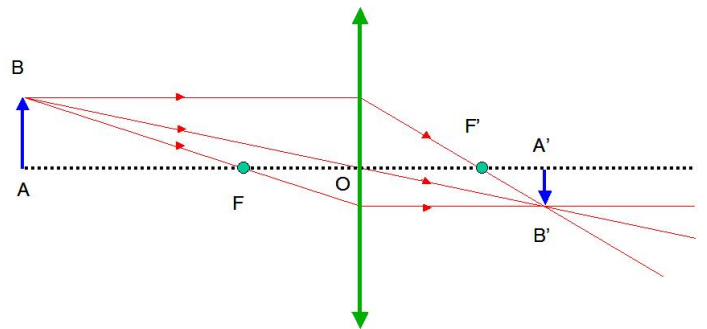
Objet situé à une distance d > 2 OF de la lentille
